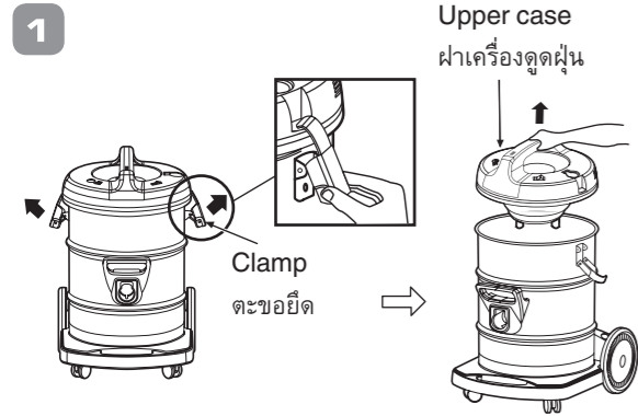
Figure shown is a vacuum cleaner Model CV-960Y ภาพที่แสดงเป็นเครื่องดูดฝุ่นรุ่น CV-960Y
