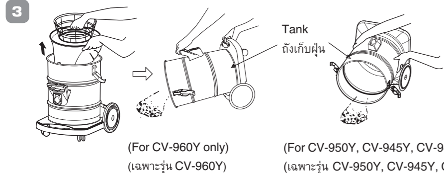
Figure shown is a vacuum cleaner Model CV-960Y ภาพที่แสดงเป็นเครื่องดูดฝุ่นรุ่น CV-960Y
